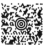
MaxiCode
